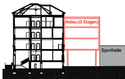
Schemat. Schnitt 1:500
