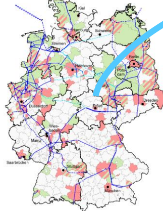
FNB H 2 -Kernnetz
